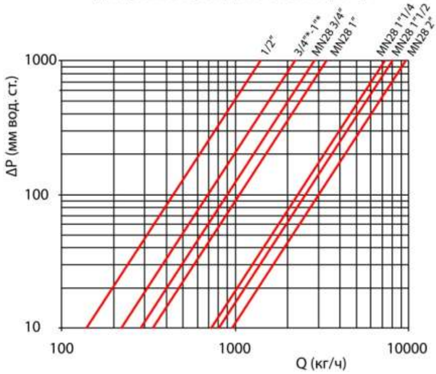
Диаграмма перепада по нефти (вязкость ≤3°E)
